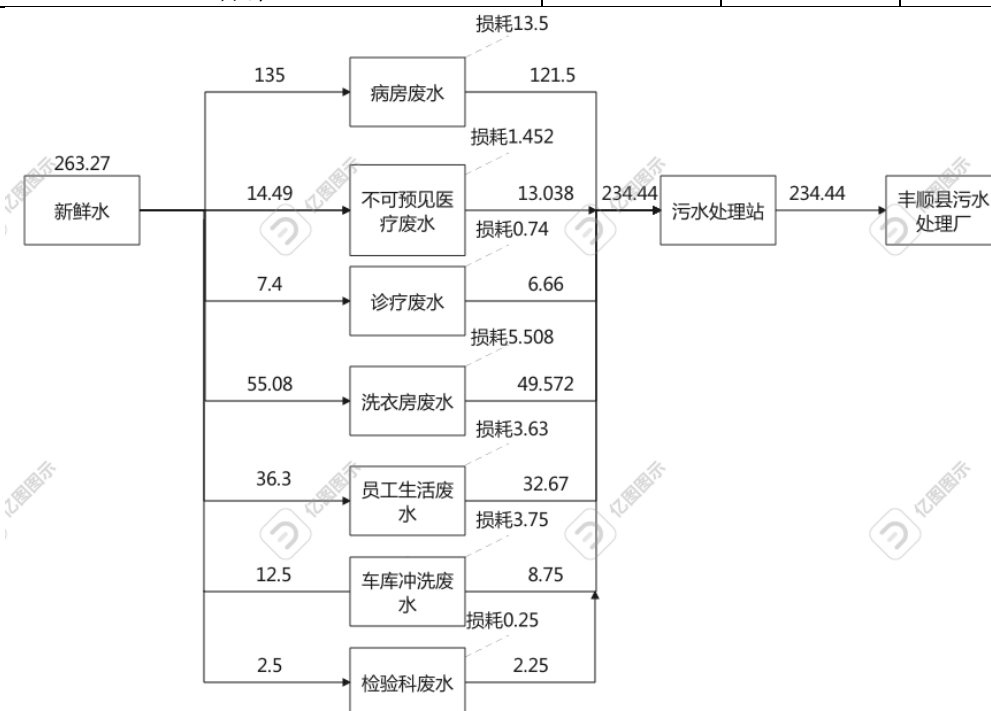
图 2-1 医院现有工程水平衡图 单位：m 3 /d
